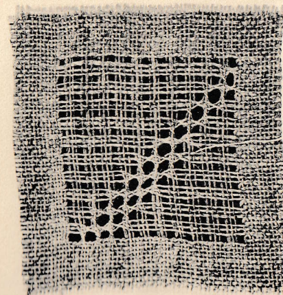
Fig. 9. Tredje varvet. När halva rutan är färdig, sys andra hälften på samma sätt.
